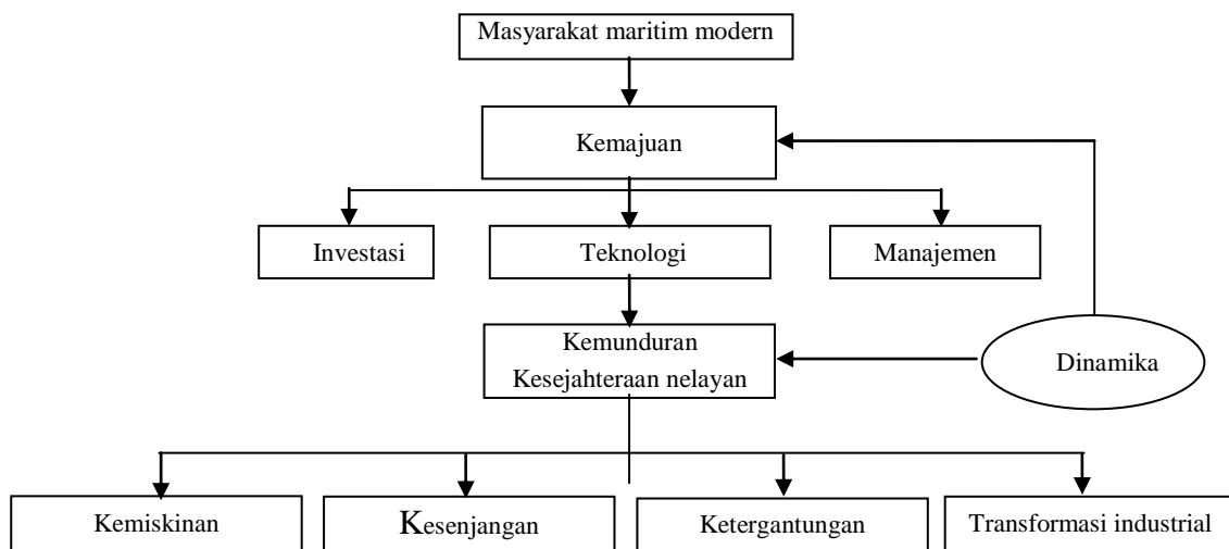
Gambar 1.1 Kerangka penelitian
